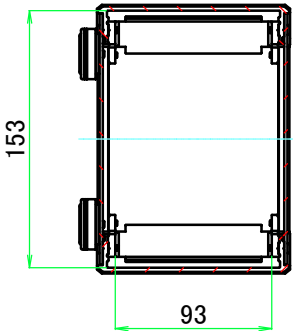
B-B ( 1 : 4.5 )
